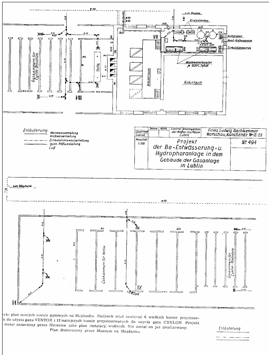
Dokument 33: Projekt der Be- und Entwässerung u. Hydrophoranlage in dem Gebäude der Gasanlage in Lublin. Undatierte Zeichnung der Firma Ludwig Reckemmer. Quelle: Z. Łukaszkiewicz, »Obóz koncentracyni i zagłady Majdanek« (siehe Dokument 6), unnummerierte Seite.
